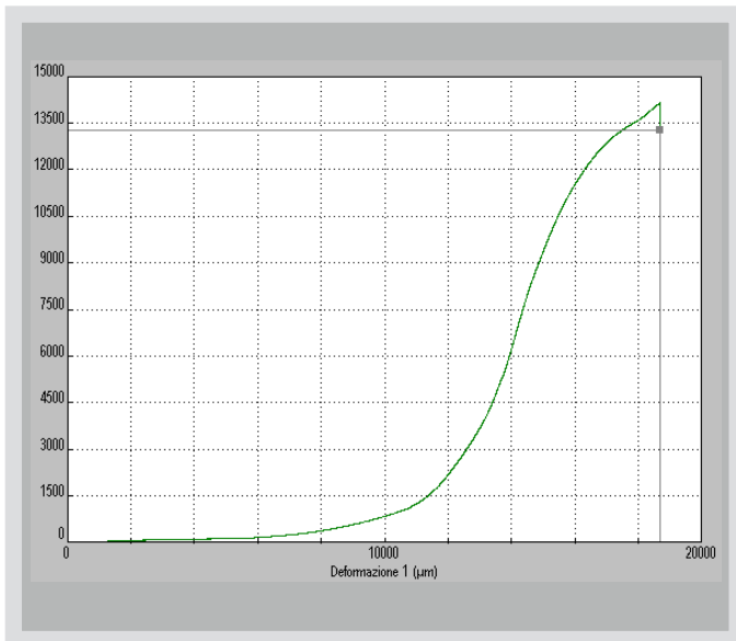
Grafico K1 basculante
