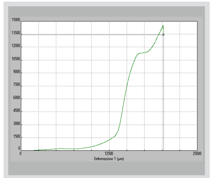
Grafico K1 fisso
